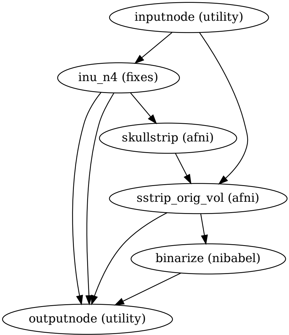
AFNISKullStripWorkflow
