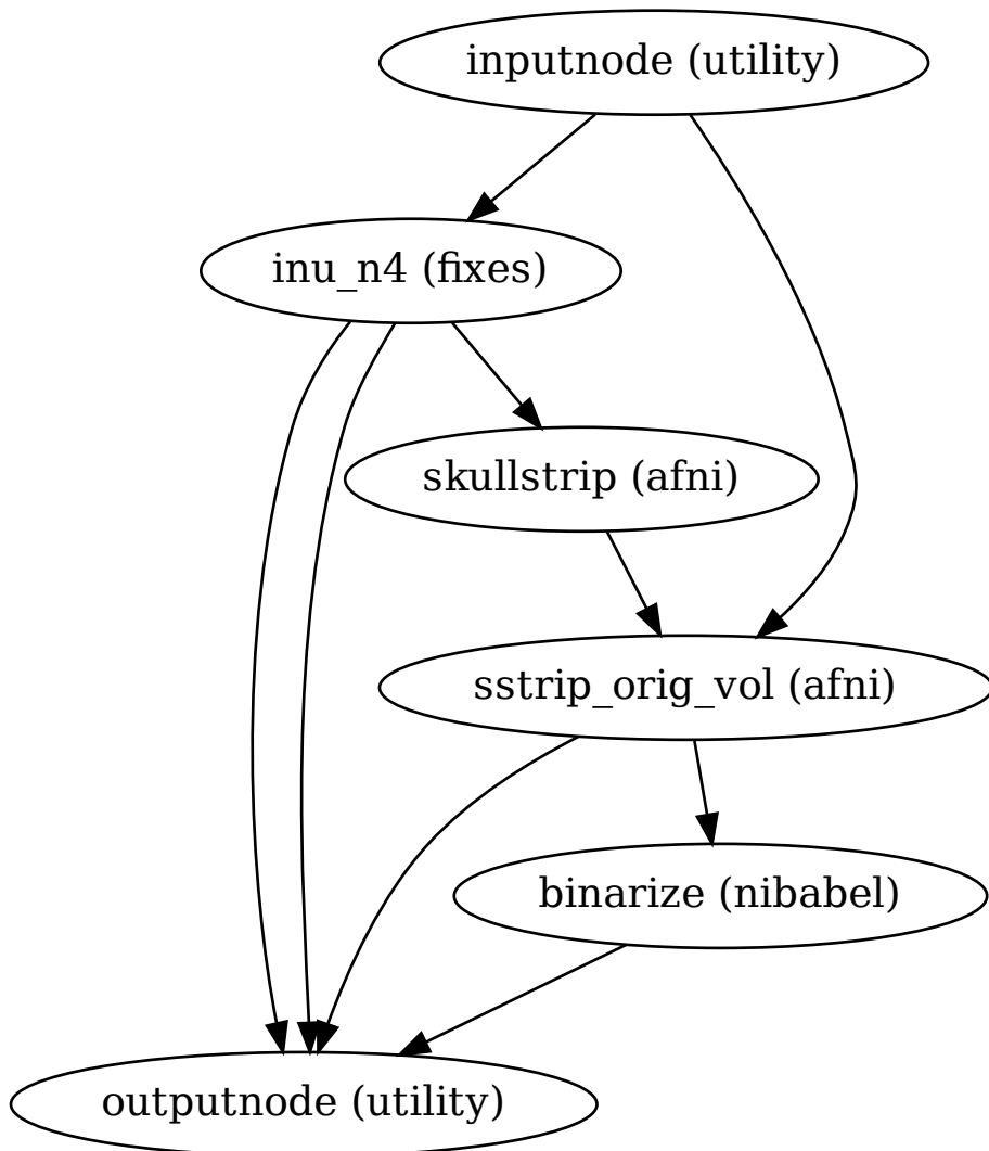
AFNISKullStripWorkflow
